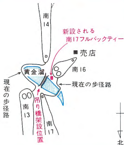
架設された黄金溜の橋梁
